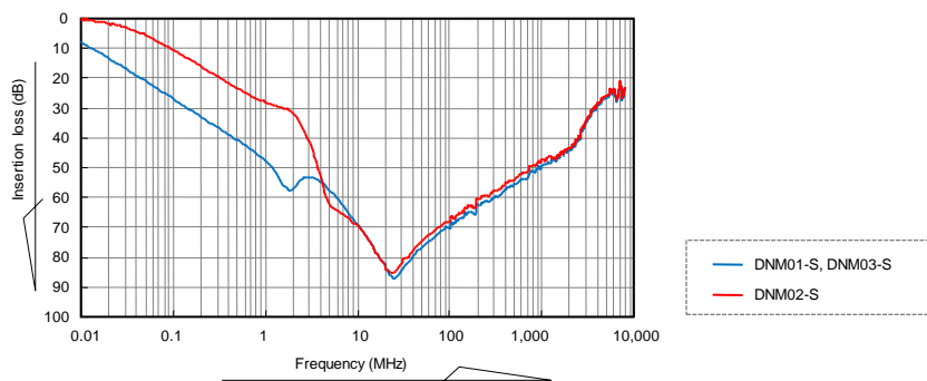
挿入損失特性
