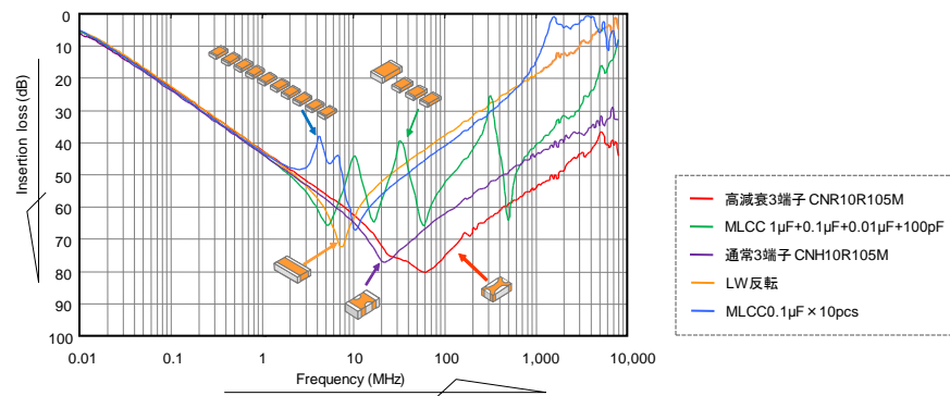
挿入損失特性(参考)
