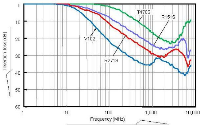
挿入損失特性(参考)
