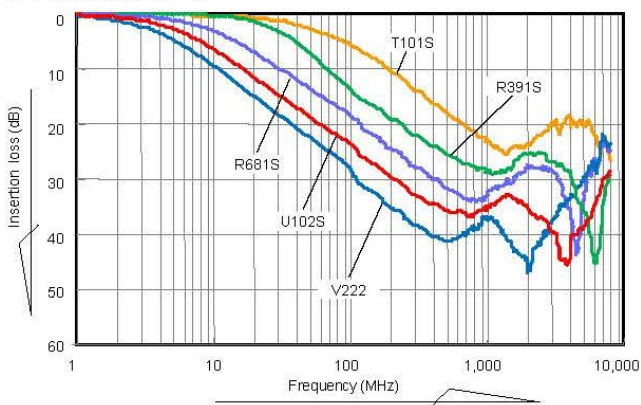
挿入損失特性(参考)
