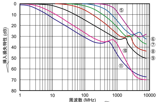
FTA30, 35タイプ挿入損失特性データ
