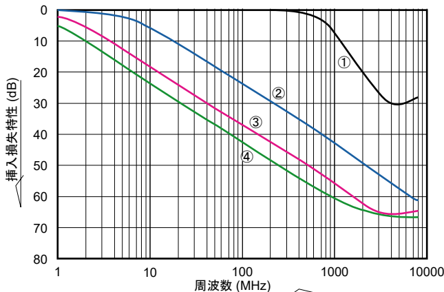
FTA30, 35タイプ挿入損失特性データ
