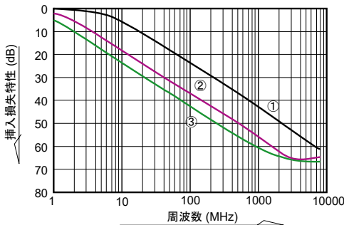
FTA322Aタイプ挿入損失特性データ
