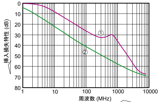
FTA41タイプ挿入損失特性データ
