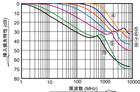
FTA322Eタイプ挿入損失特性データ
